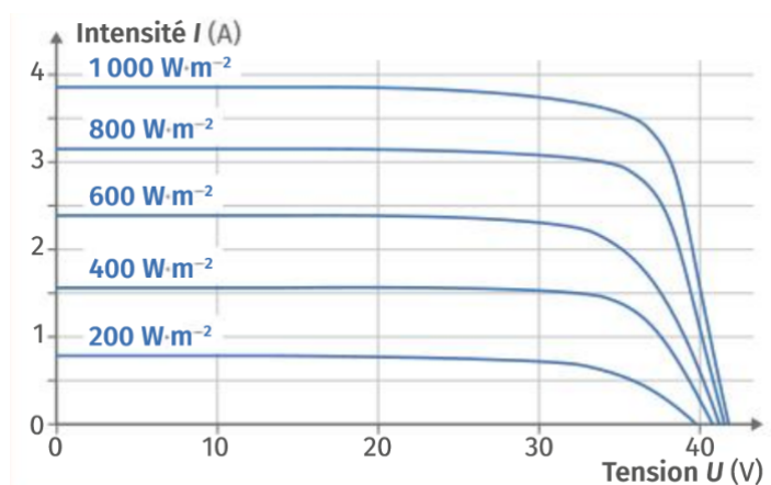
Document 1 : Caractéristiques intensité-tension
